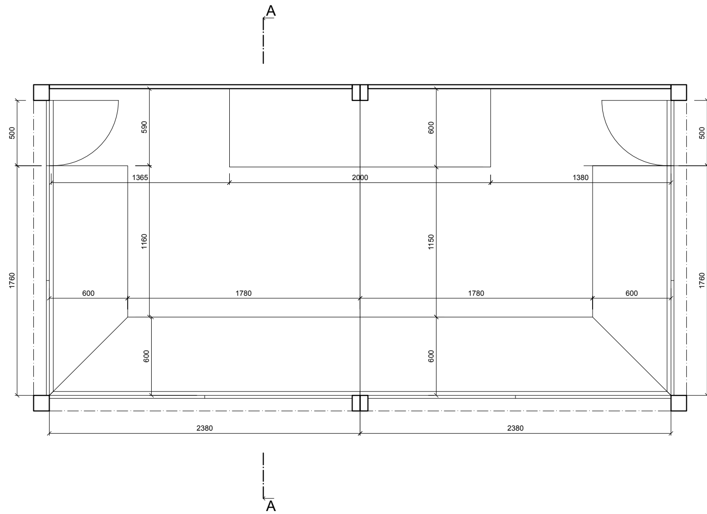
BAR - PŮDORYS KONSTRUKCE CELKOVÁ PLOCHA BARU = 10,9m 2
